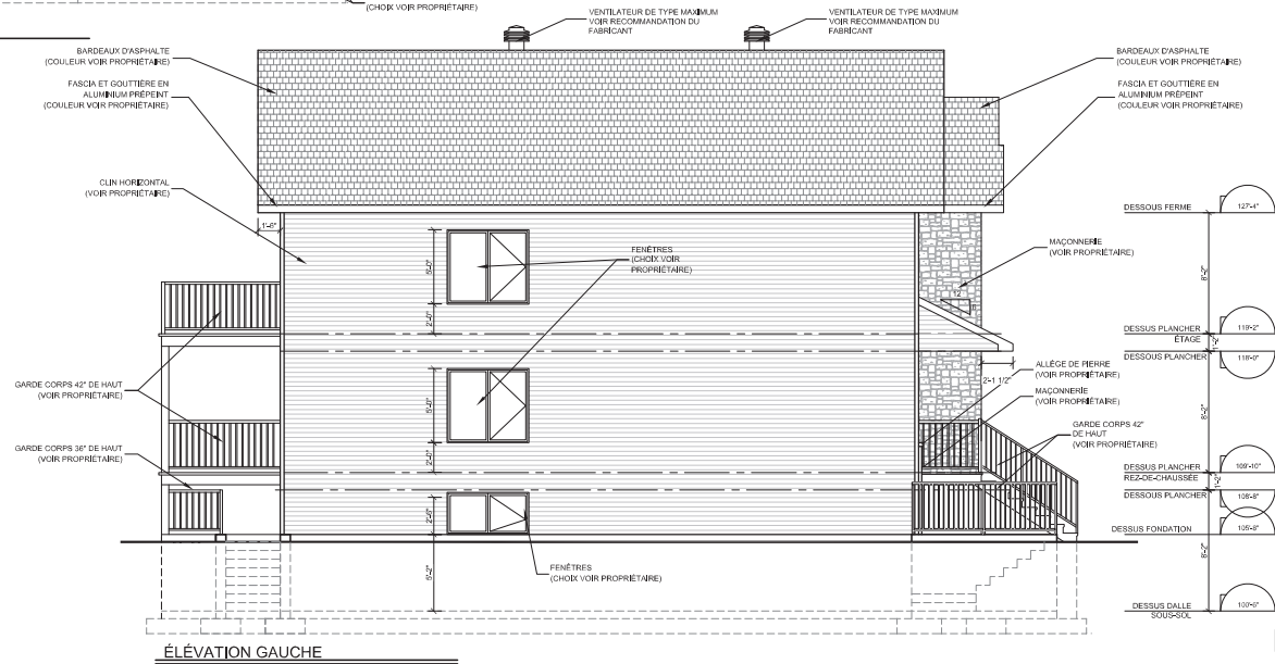
ÉLÉVATION GAUCHE
